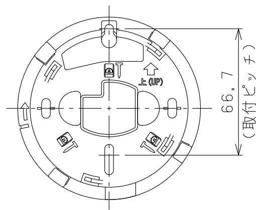
取付寸法図
